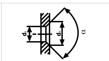
Pulttinreiän rakenne - kartiomainen
